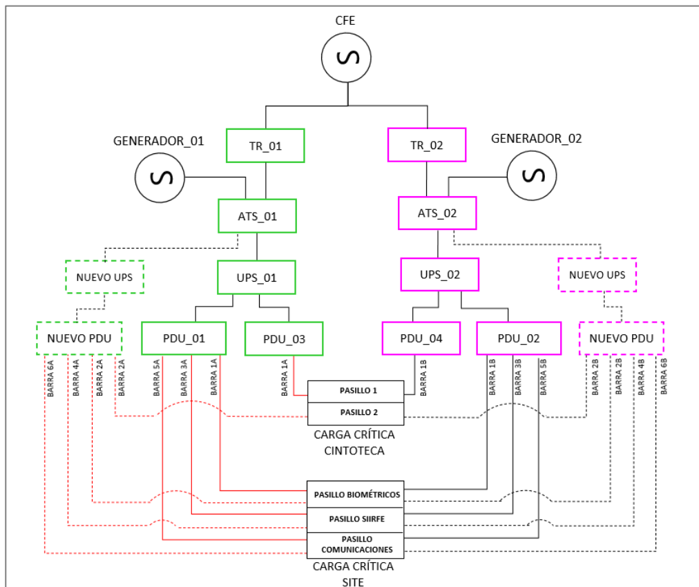
Diagrama 2: Configuración eléctrica final del CCP.
