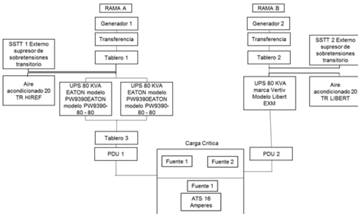
Diagrama 1: Configuración eléctrica actual del CCS.
