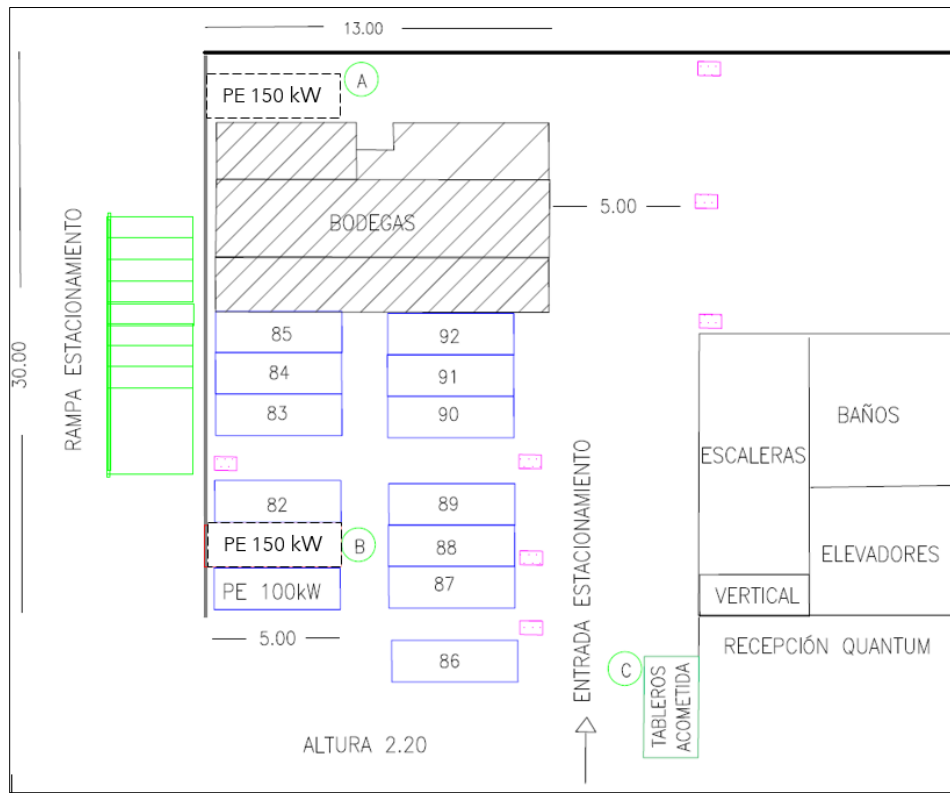
Diagrama 2. Ubicación de las plantas de emergencia en Planta Baja (estacionamiento) del Edificio de Quantum.
