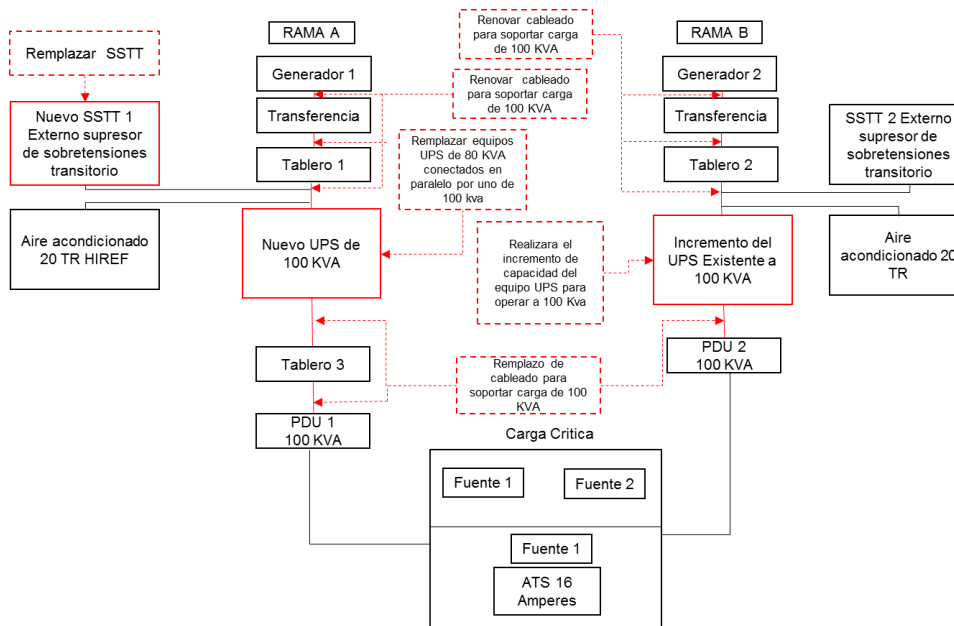
Diagrama 3: Nueva configuración eléctrica del CCS
