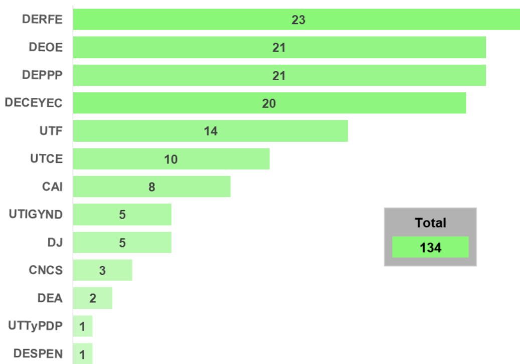
Gráfica 4 Distribución absoluta del total de actividades en tiempo por UR del PlyCPEF 2023-2024
