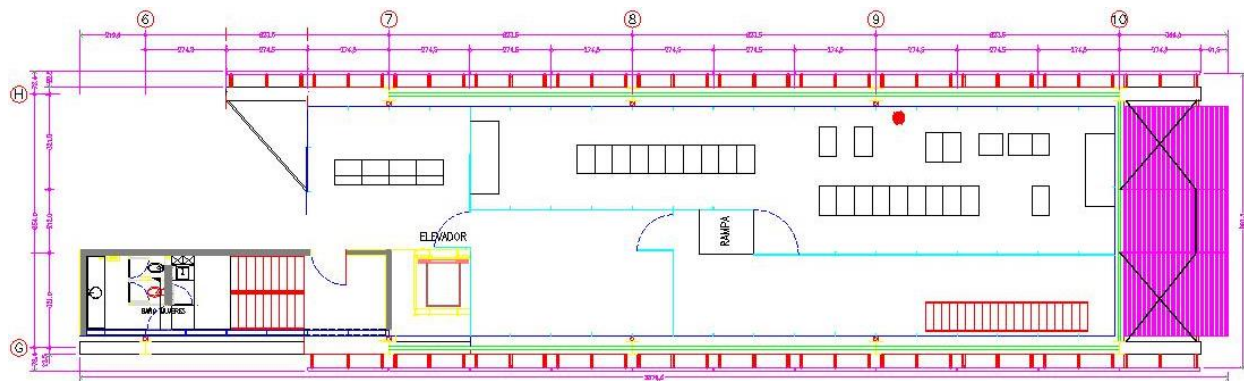
Figura 8: Piso 4
