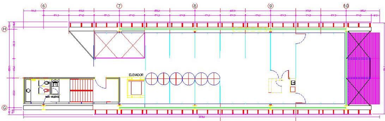
Figura 6: Piso 2
