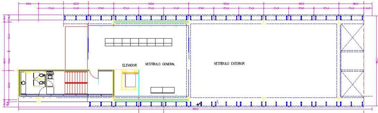
Figura 4: Planta baja
