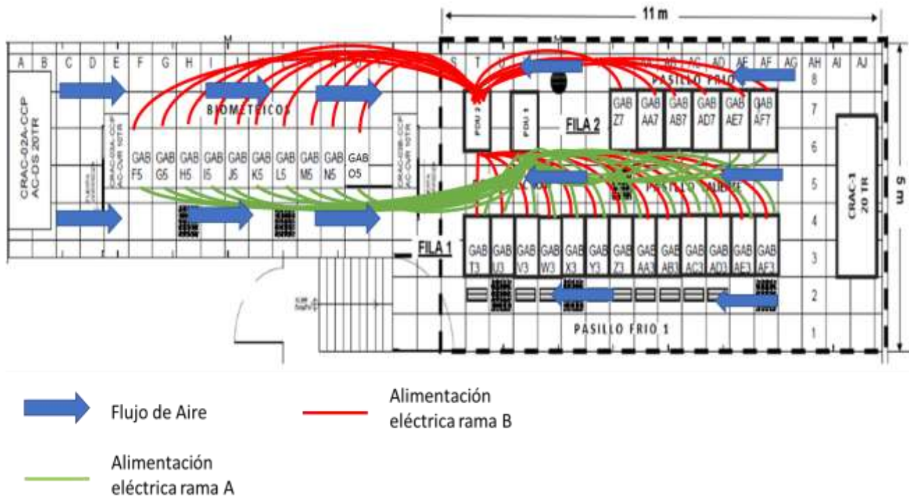
Diagrama 1: Configuración Alimentación Eléctrica actual del CCP.
