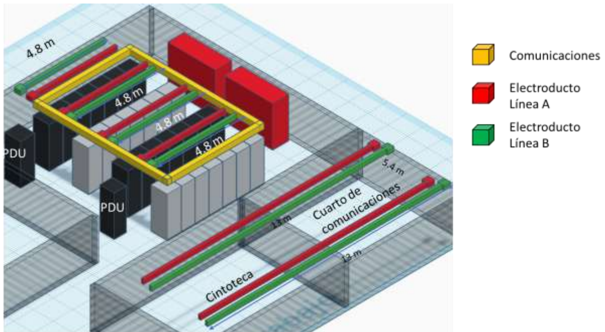
Diagrama 4: Alimentación eléctrica por Electroducto del CCS
