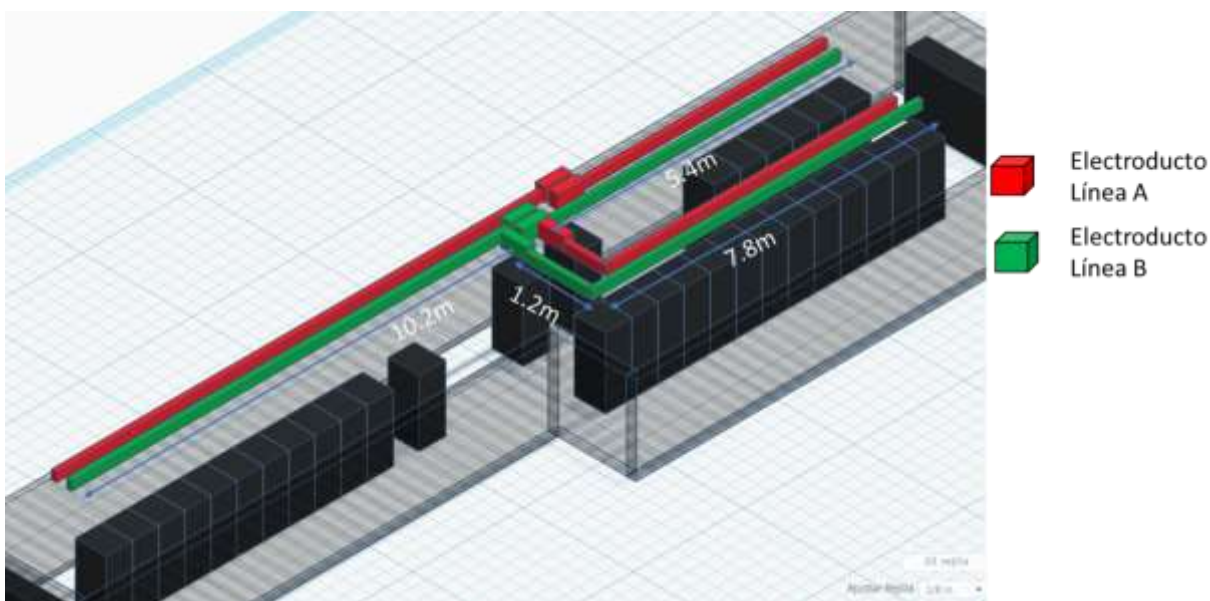
Diagrama 3: Alimentación eléctrica por Electroducto del CCP
