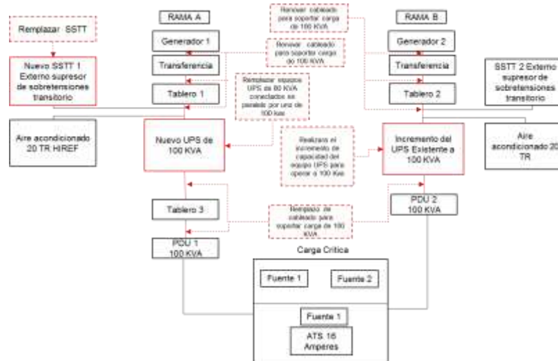
Diagrama 3: Nueva configuración eléctrica del CCS
