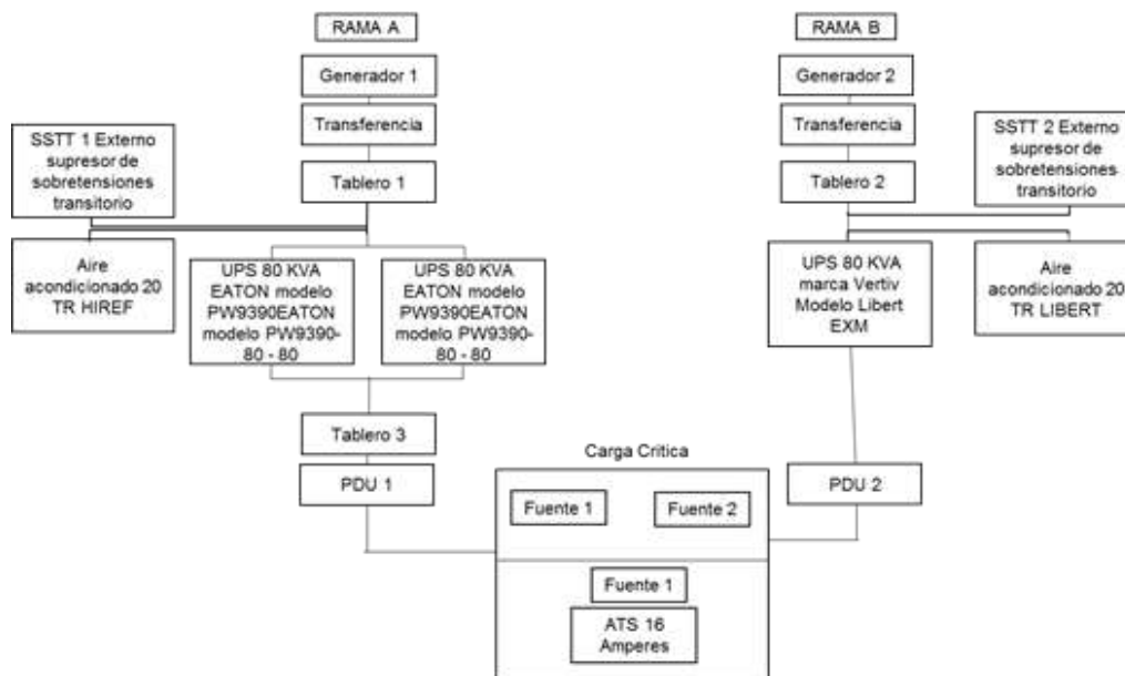
Diagrama 1: Configuración eléctrica actual del CCS.
