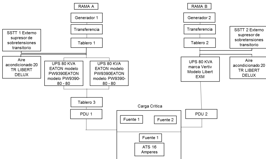
Diagrama 1: Configuración eléctrica actual del CCS.
