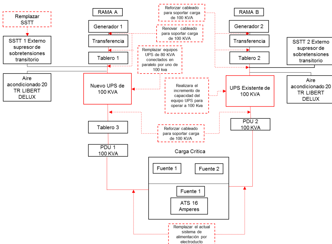
Diagrama 3: Nueva configuración eléctrica del CCS
