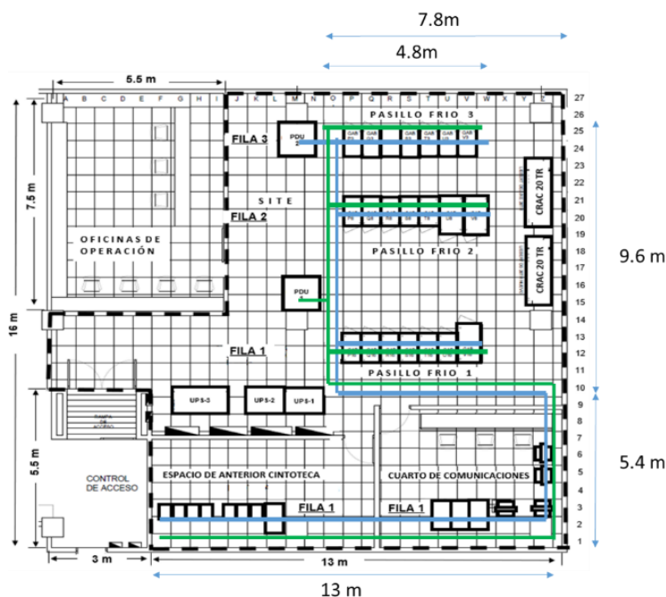
Diagrama 4: Alimentación eléctrica por Electroducto del CCS
