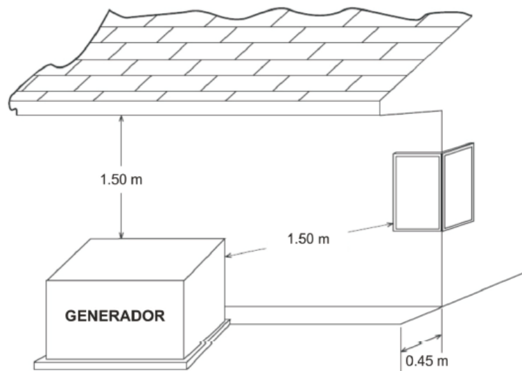
Ilustración 2 - Lugar para la instalación del Generador
