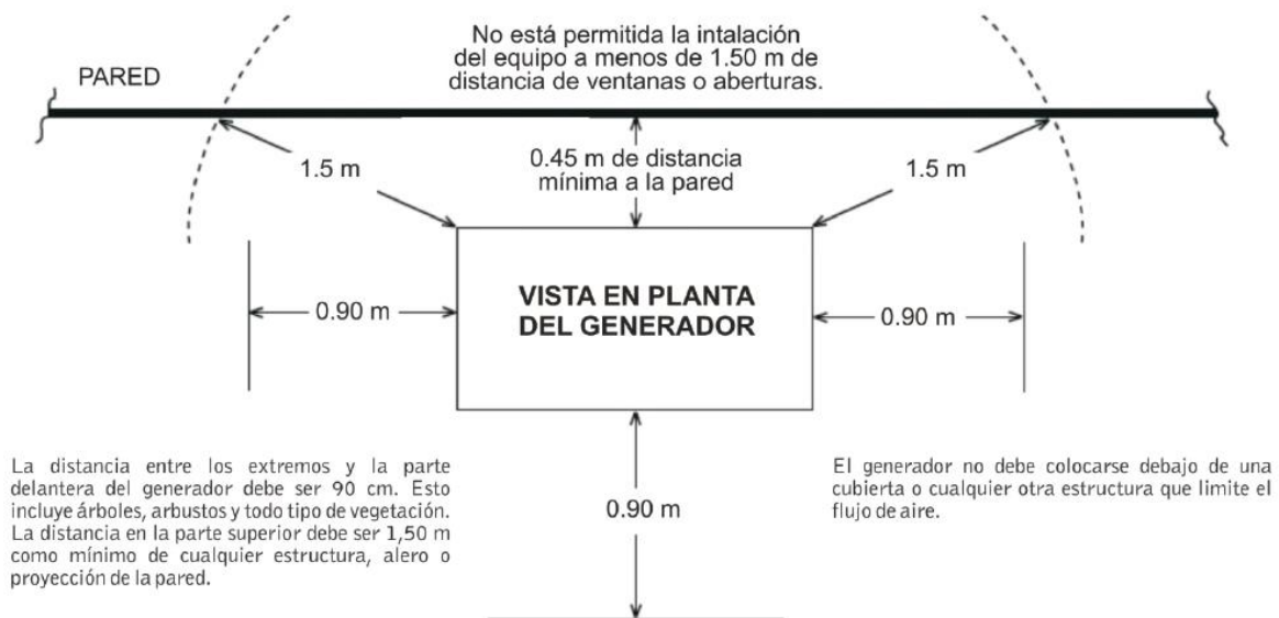
Ilustración 1 - Distancias para la instalación del Generador
