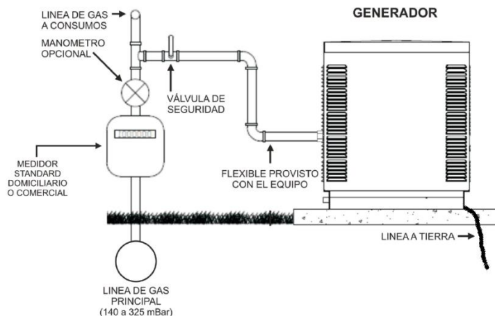
Ilustración 3 - Diagrama de instalación de línea de gas
