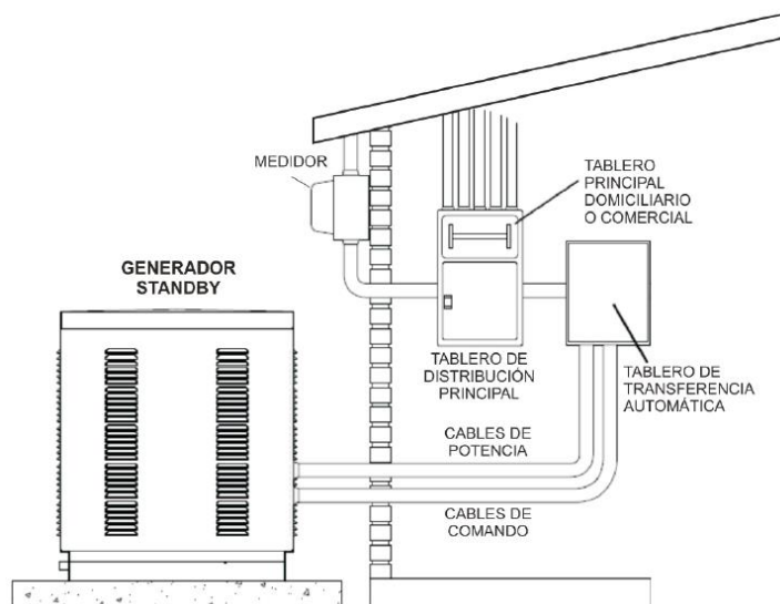
Ilustración 4 -Diagrama general de la instalación
