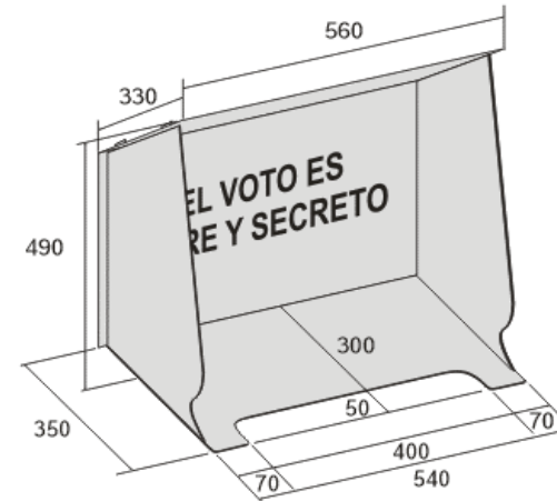
ISOMÉTRICO
