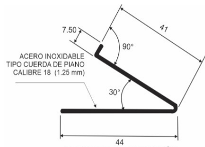
RESORTE DE PIN BOTÓN ACOTACIONES EN MILÍMETROS
